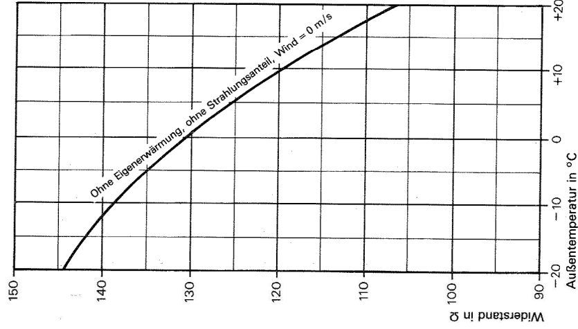
Außentemperatursensor, Best.-Nrn. 7401 990 und 9580 177
