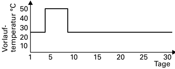
Temperatur-Zeit-Profil 2 (F1:2)
