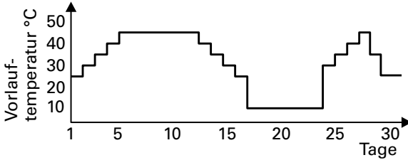
Temperatur-Zeit-Profil 3 (F1:3)
