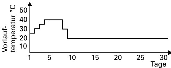
Temperatur-Zeit-Profil 4 (F1:4)
