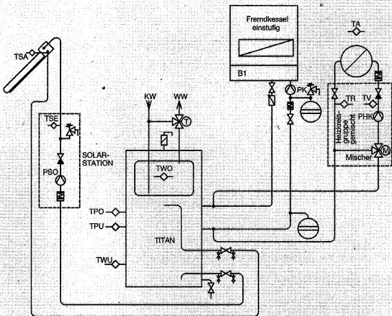
Abbildung 2: Anschlusschema TITAN Aqua
