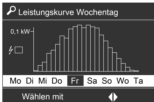
Abb. 37 Für jede Stunde eines Tags wird 1 Balken angezeigt. Die Balkenhöhe gibt die gemittelte elektrische Leistung über 1 h an.
