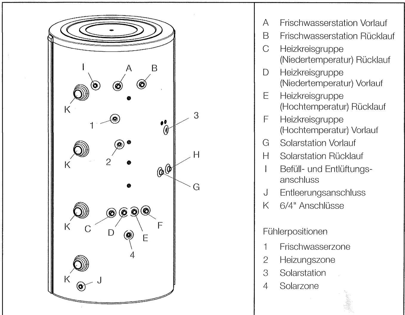
Bild 11: Aufbau des Systemspeichers
