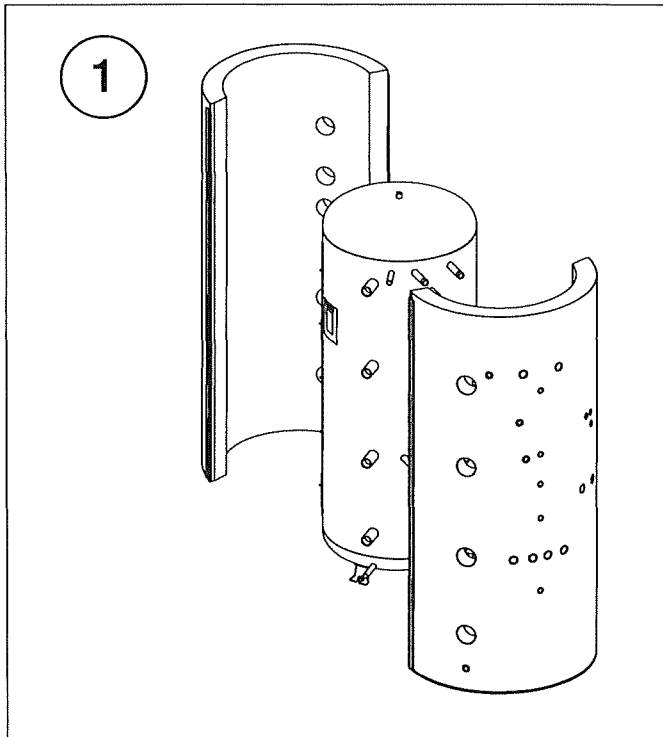
Bild 12: Isolierung aufbringen
