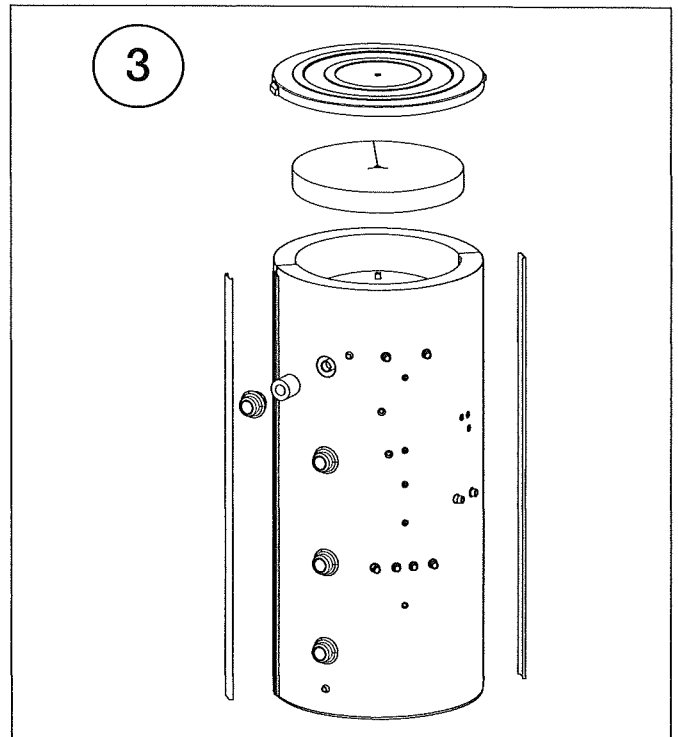
Bild 14: Klemmleisten-Abdeckung, Weichschaumring, Tiefziehdeckel, Schaumstoffrossetten und Isolierkappen aufbringen
