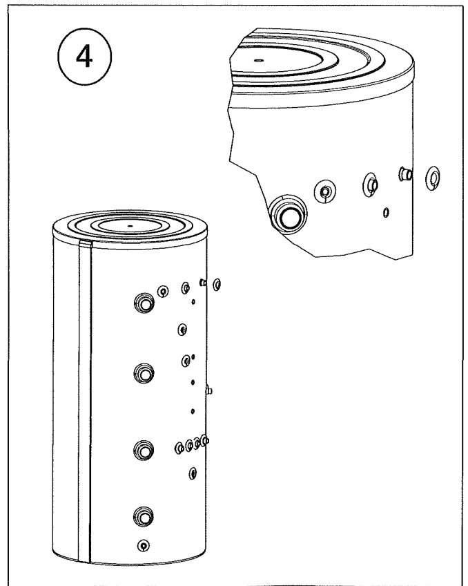
Bild 15: Kunststoffrossetten aufstecken
