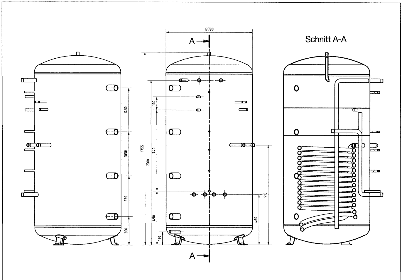
Bild 16: Abmessungen des FWSS 800
