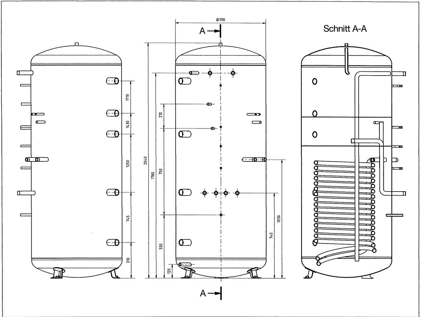
Bild 17: Abmessungen des FWSS 1000
