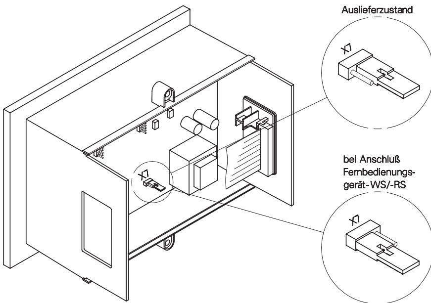
(A) Fernbedienungsgerät-WS/-RS
