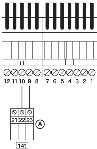
Ⓐ Stecker 141 zum Anschluß an Erweiterungssatz
