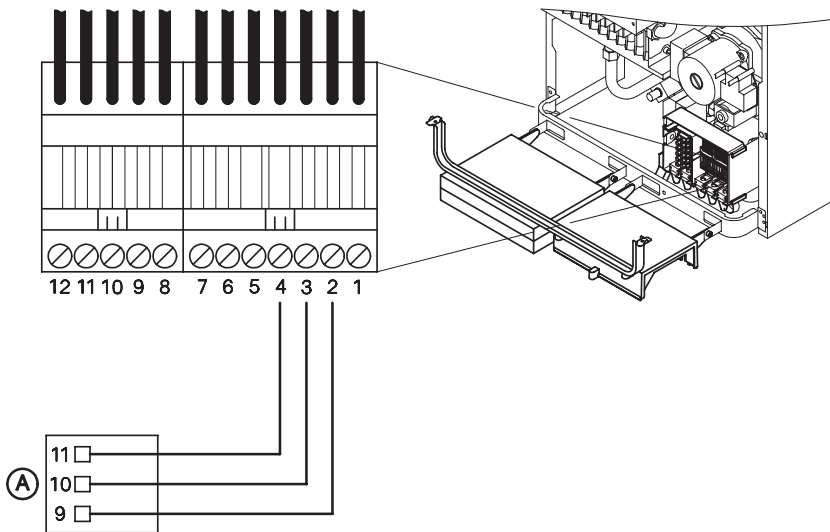
(A) Fernbedienungsgerät-WS/-RS
