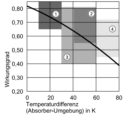
Vitosol 200-F, Typ SV2D
